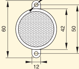
CTR4-RFL000014 Spessore 6 mm Thickness 6 mm
