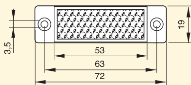
CTR10-RFL000018 Spessore 9,5 mm Thickness 9,5 mm
