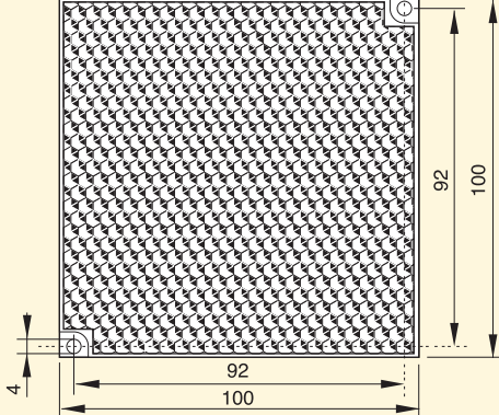
CTR10-RFL000018 Spessore 9,5 mm Thickness 9,5 mm
