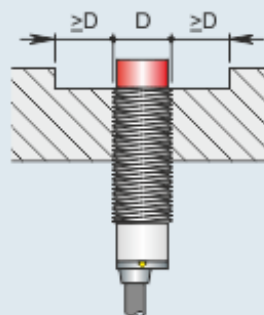
Montaggio sporgente
