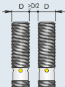
Montaggio affiancato
