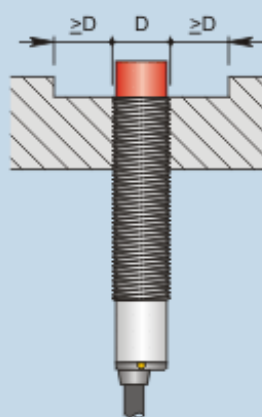
Montaggio sporgente
