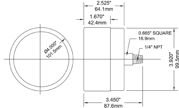
Conexión Posterior de Latón de 4"
