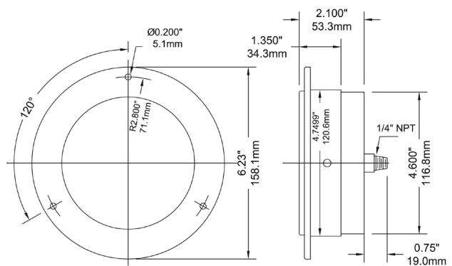
Conexión Posterior de Acero Inoxidable con Pestaña Frontal de 4.5"
